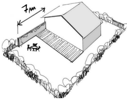
Exemples de murs sur l'arrière des façades
